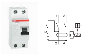
Серия FH200
